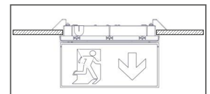
Χωνευτή τοποθέτηση με εξαρτήματα στήριξης και πινακίδα σήμανσης
