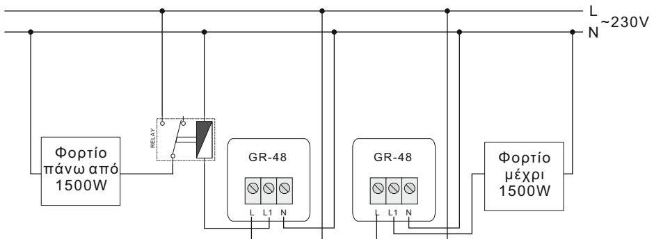
Συνδέσεις GR-48
