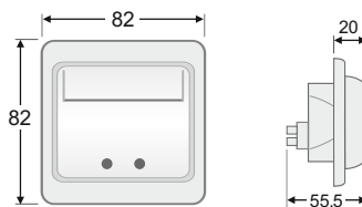
Διαστάσεις RF-53/A σε χιλ.
